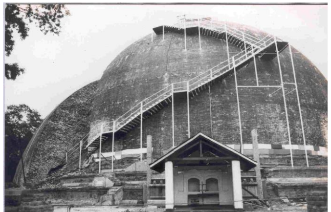
修復後のミリスアウェティヤ仏塔ドームの崩壊：1980 年代の 2 回目の試み
