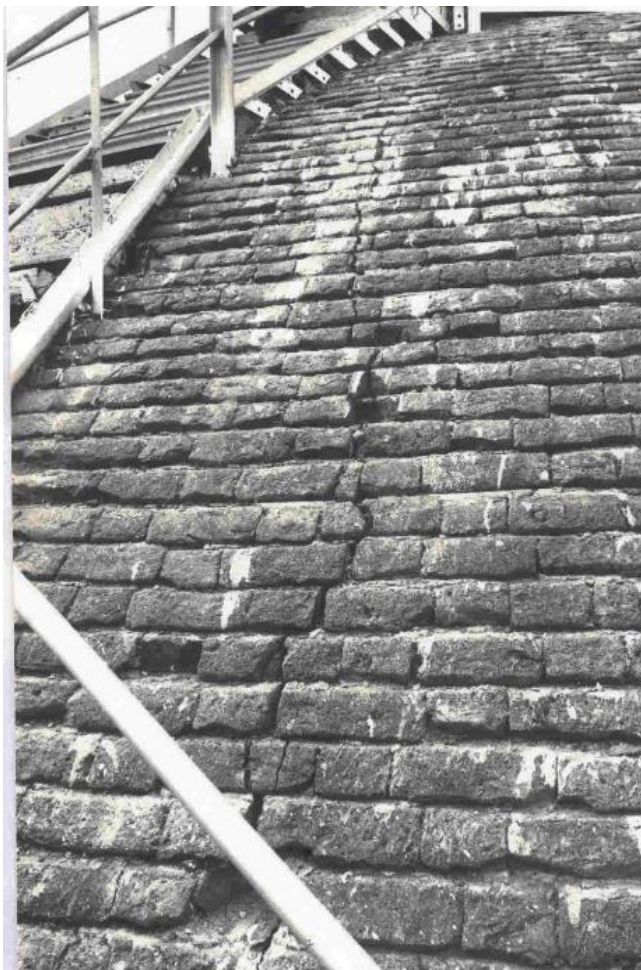
崩壊前のミリスアウェティ仏塔ドーム上の亀裂
