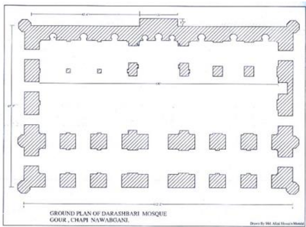
ダラスバリ・モスクの平面図
